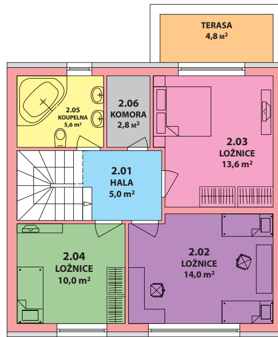
2.NP
