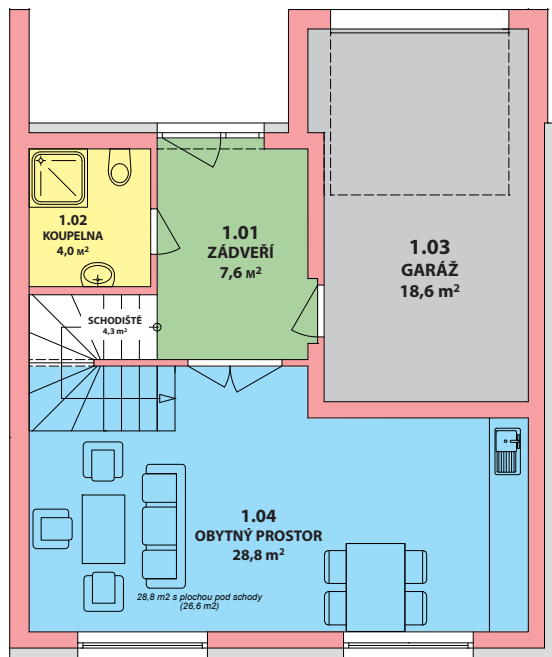
1.NP
